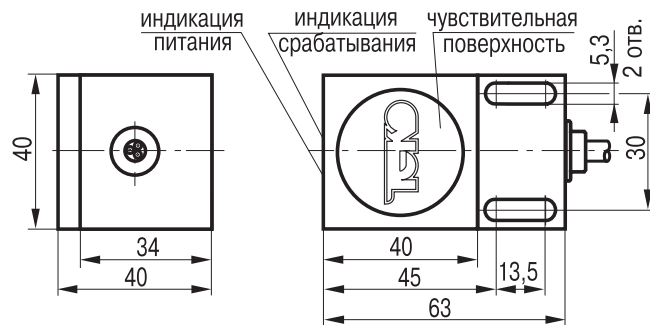
Габаритный чертеж
